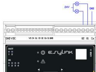
Figure 3 : Exemple de branchement des sorties
